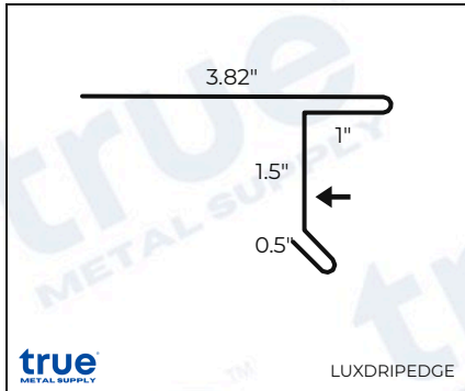
Drip Edge
